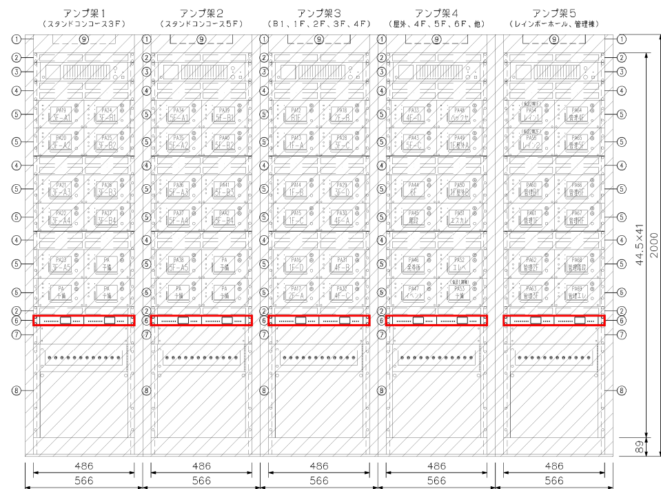
正面图
