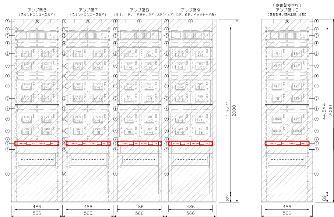
正面图
