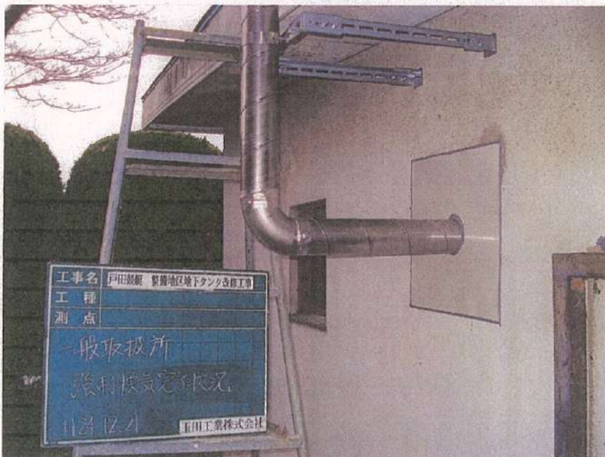
一般取扱所工事 強制換気交換工事 完了状況 外部
