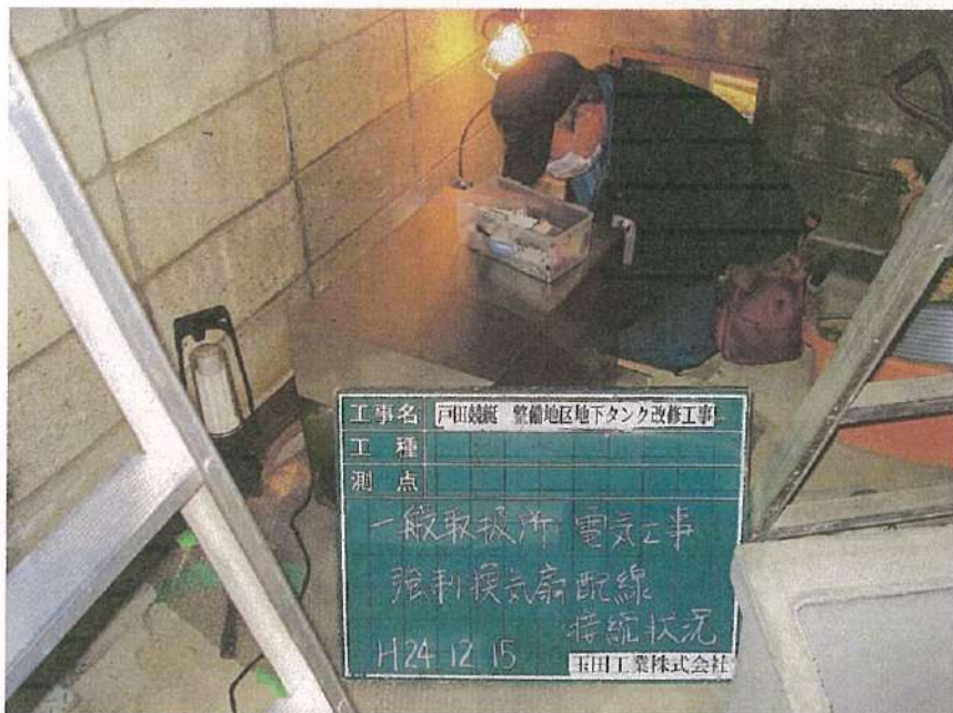
一般取扱所工事 強制換気交換工事 電気結線状況
