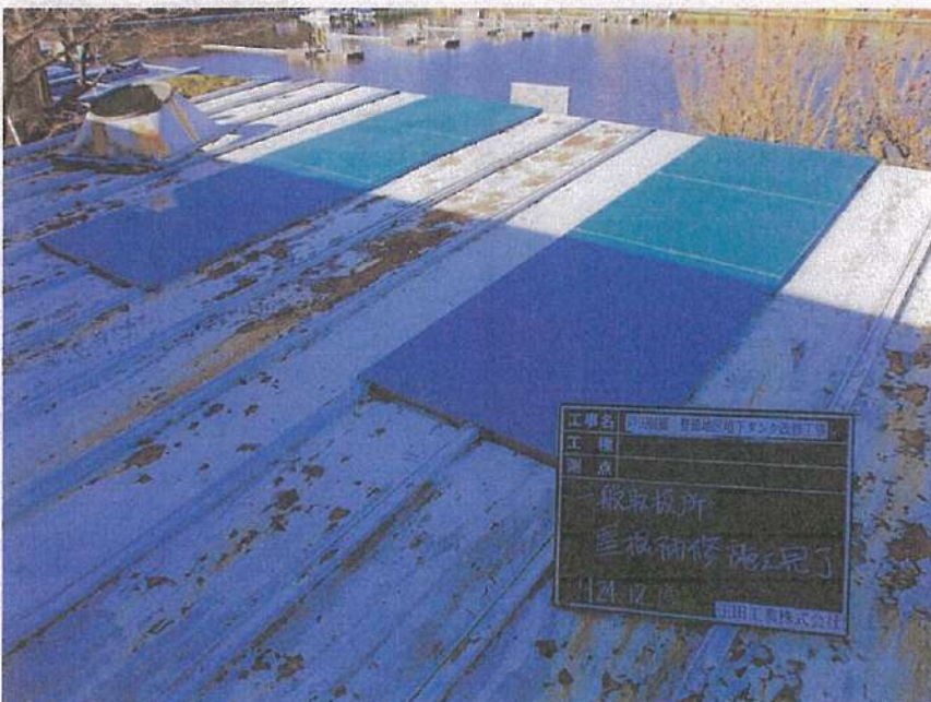
一般取扱所工事 屋根上換気塔 撤去工事 屋根復旧状況 屋根材張り完了
