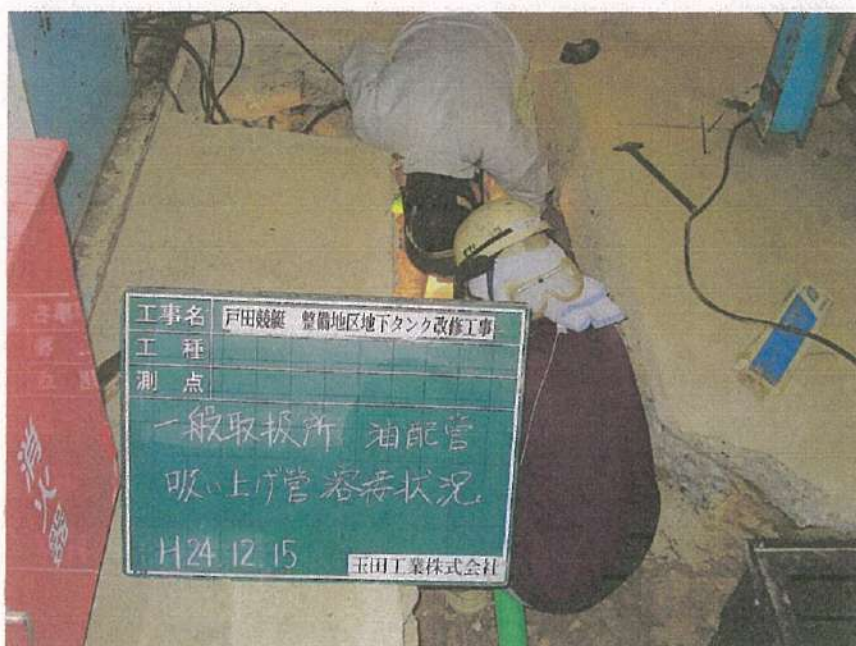
一般取扱所工事 油配管工事 吸上げ管溶接状況
