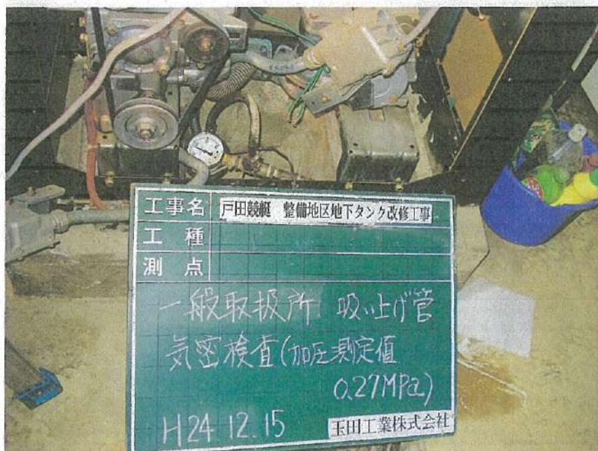
一般取扱所工事 油配管工事 吸上げ管気密検査 (加圧測定値：0.27MPa)
