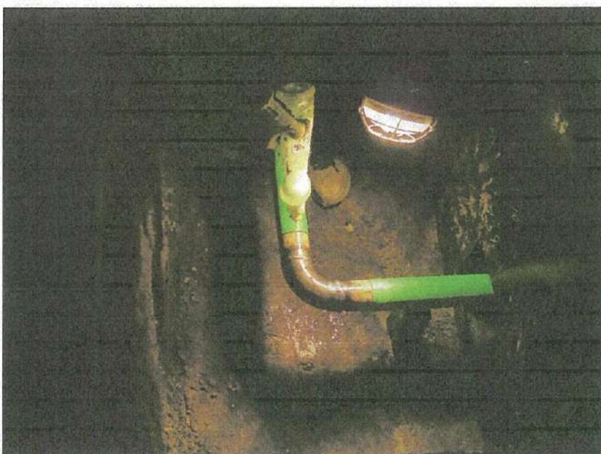
一般取扱所工事 油配管工事 自主検査 発砲検査状況
