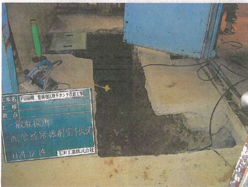
一般取扱所工事 解体工事 配管経路 掘削完了状況
