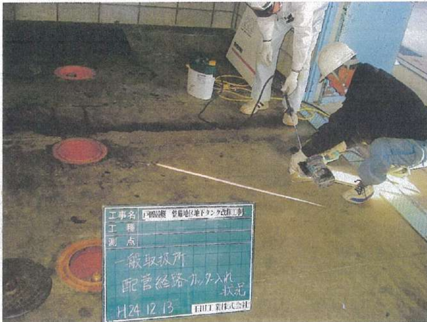
一般取扱所工事 解体工事 配管経路カッター入れ状況
