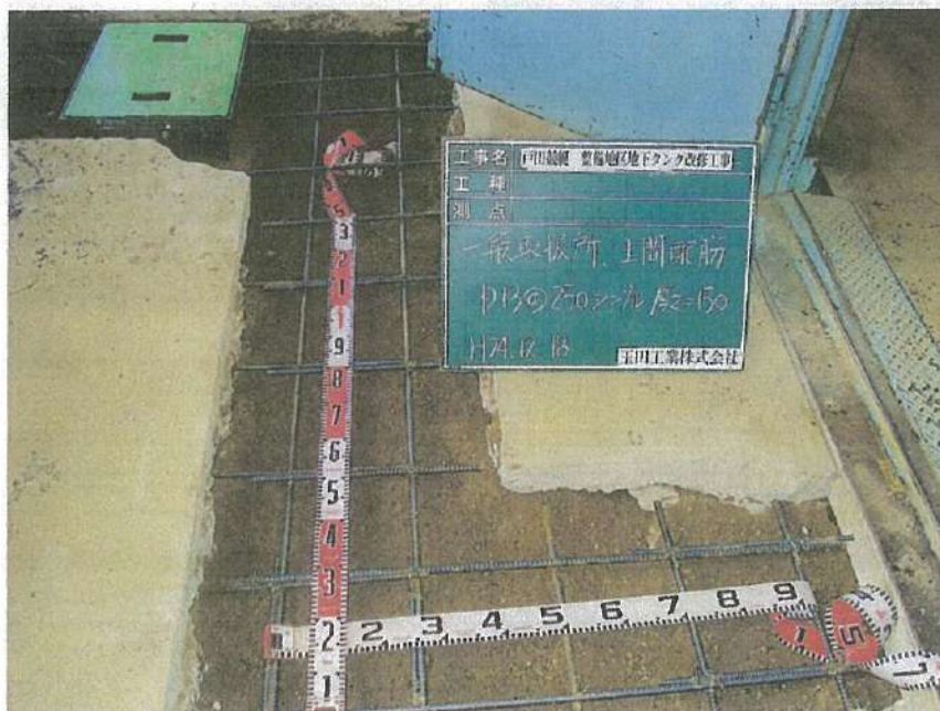
一般取扱所工事 鉄筋工事 配管経路土間 D13@250(タテ、ヨコ共) シングル 厚さ=150
