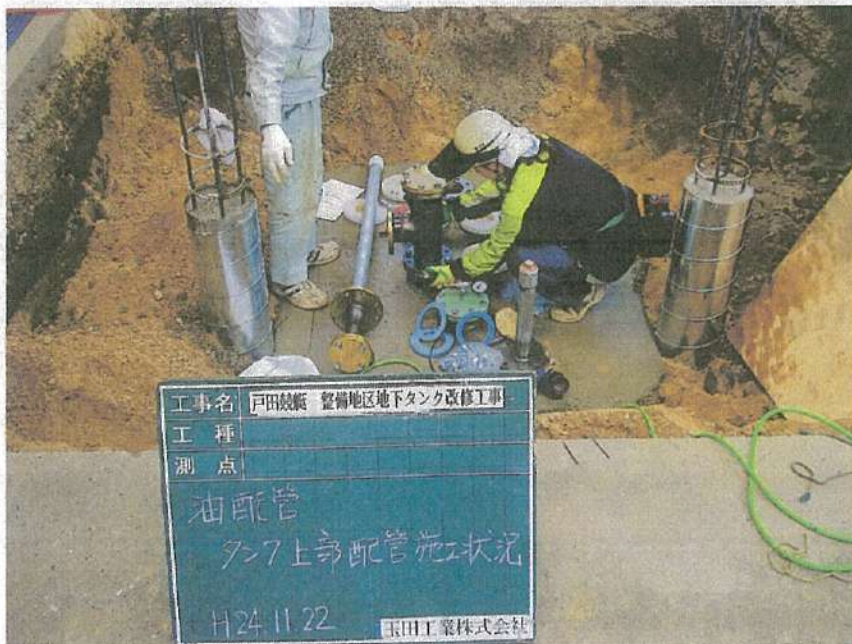
地下タンク設置工事 油配管 タンク 上部配管状況
