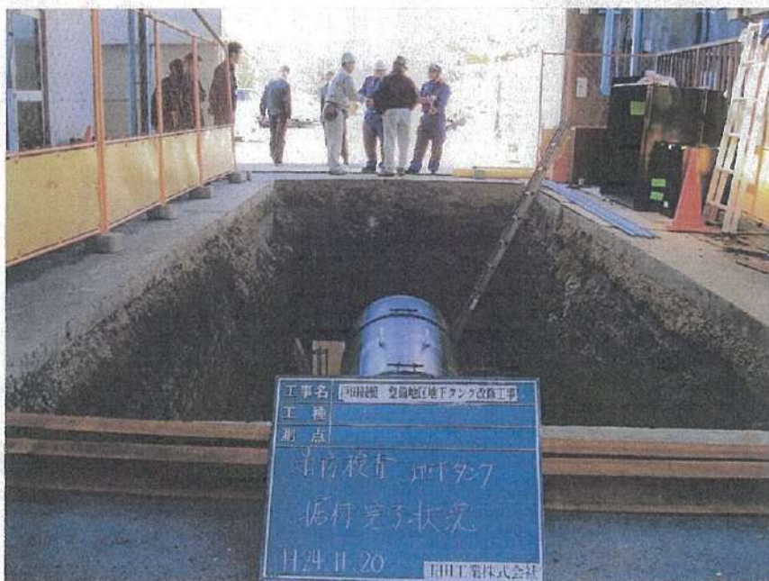
地下タンク設置工事 SF二重殻・6Kタンク 現場設置 完了状況
