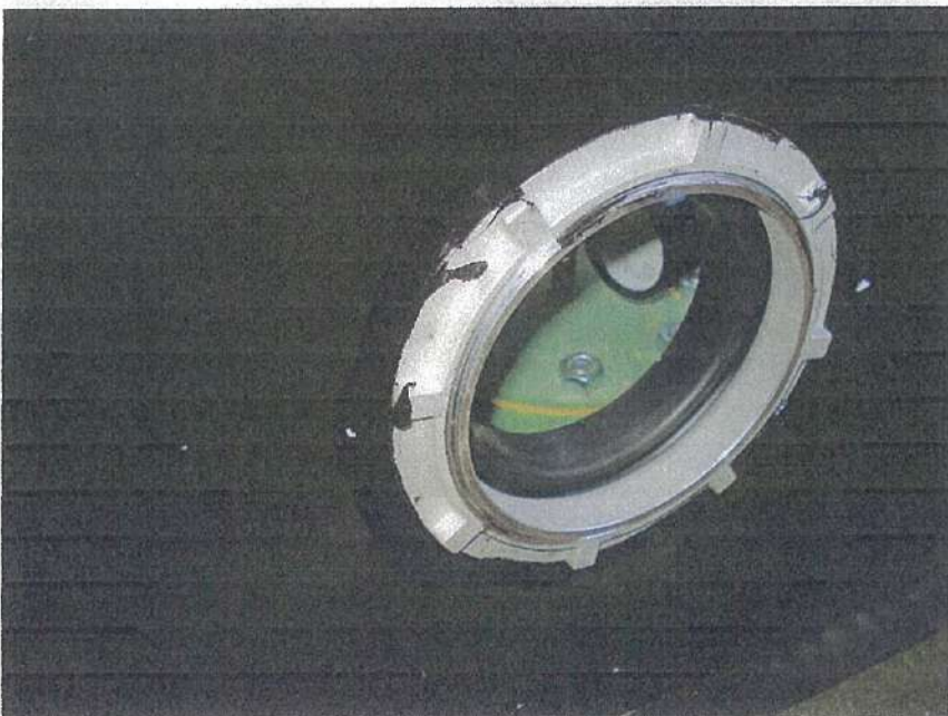
地下タンク設置工事 油配管 タンク上部配管 プロテクター貫通部 配管ソケット取付後 周囲シーリング打設 完了状況
