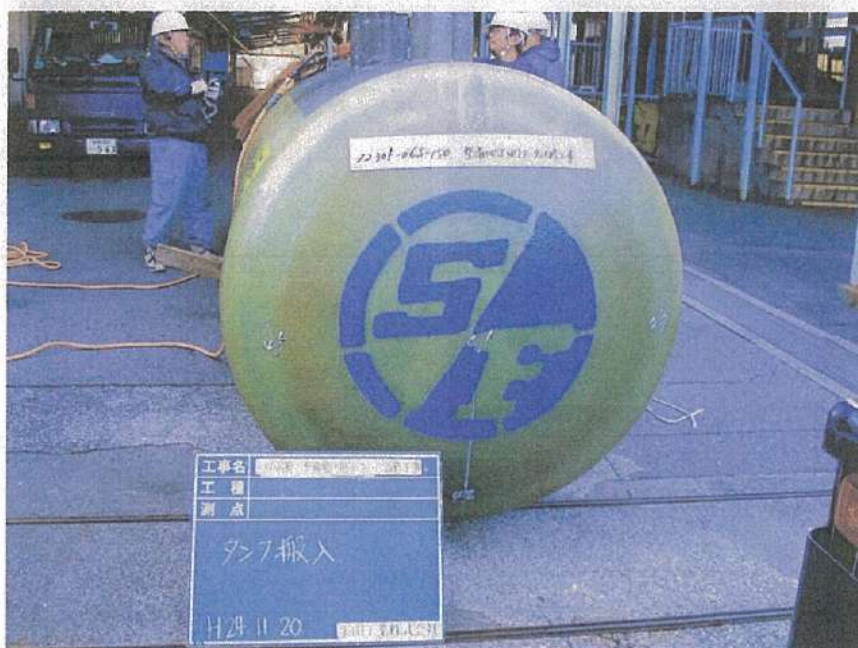
地下タンク設置工事 SF二重殻・6Kタンク 搬入状況
