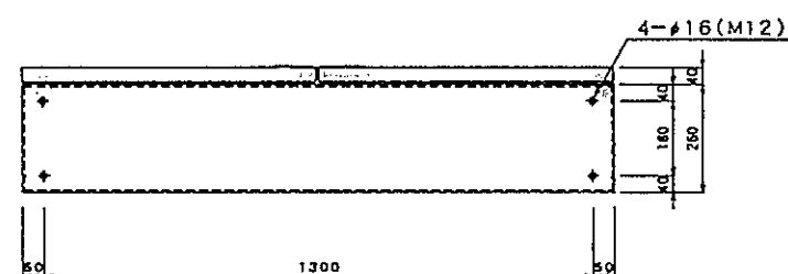
底面图
