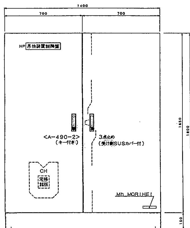
正 面 图
