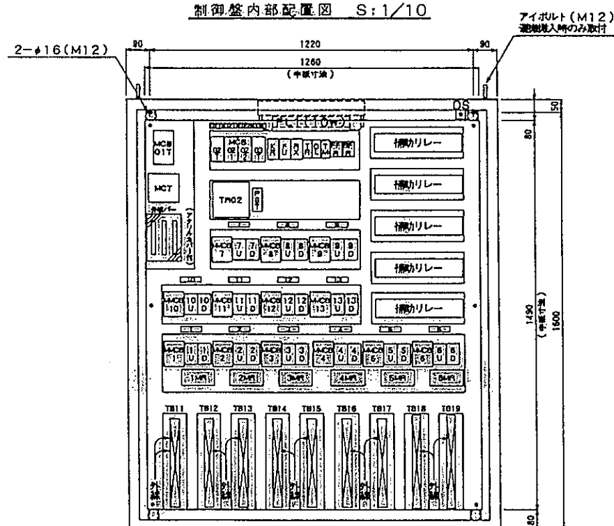
制御盤内部配置図 S:1/10
