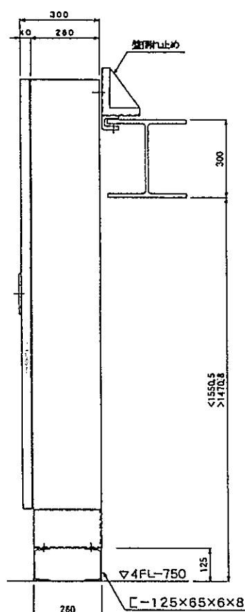
側面図
