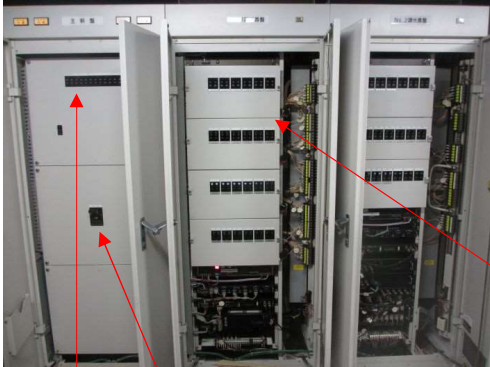
主幹盤 (既設)
